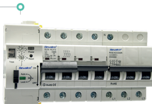
Interruptores automaticos RV30-10 KA Curva B, C y D. 4 Polos + Protector sobretensiones IGA
