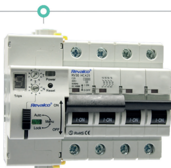
Interruptores automaticos RV30-10 KA Curva B, C y D 4 Polos
