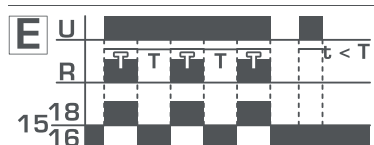
Cíclico simétrico, comienzo por impulso
